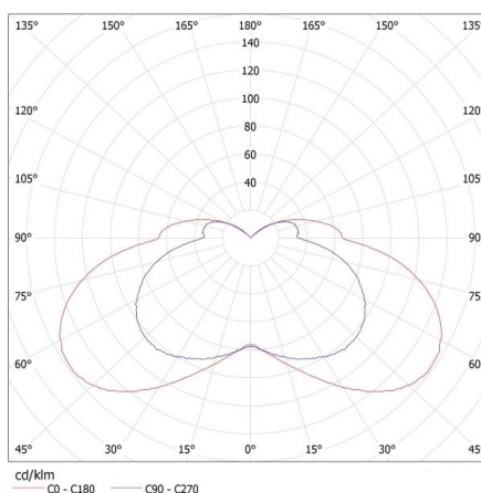
KANLUX S.A. (kat 23104) TERRA LED / Krzywa rozsytu światła (biegunowo)
